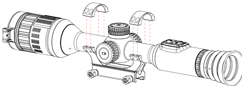
Obrázek 2-6 Umístění zařízení do prstence
