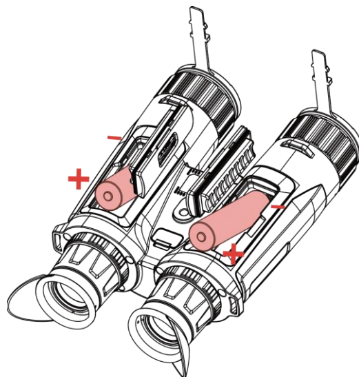
Фигура 2-2 Поставяне на батерията
