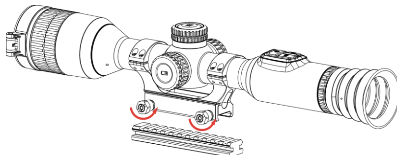
Abbildung 2-8 Schrauben lösen
