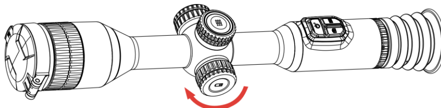
Abbildung 2-4 Abdeckung festziehen
