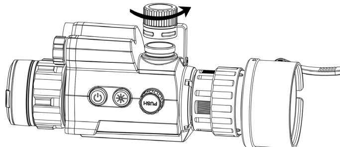
2-3 ábra Az akkumulátor fedőlapja nyitott állapotban
