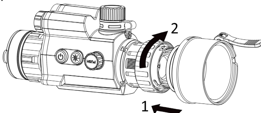
2-2 ábra Az adapter beszerelése
