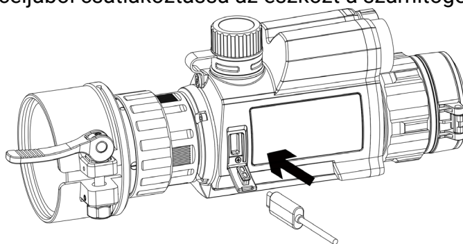
2-1 ábra Kábelcsatlakozók
