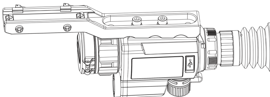
2-7 ábra Csavarok meghúzása
