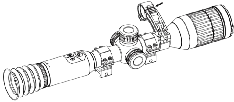
그림 2-11 레버 잠그기
