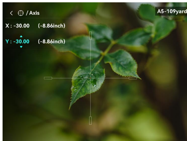
그림 4-3 레티클 보정
