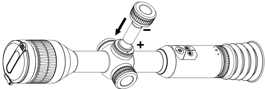
그림 2-3 배터리 설치하기
