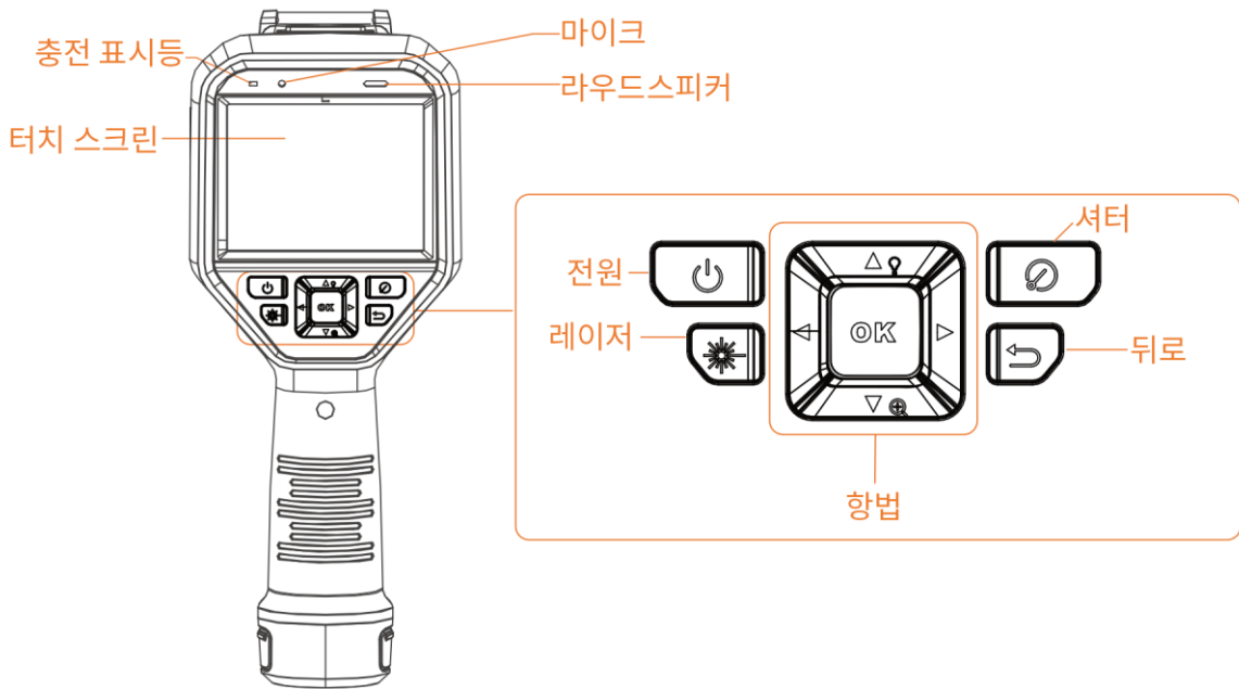
그림 1-1 외관(전면도)
