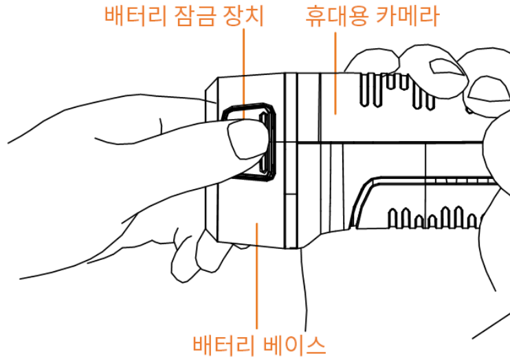
그림 2-1 배터리 분리
