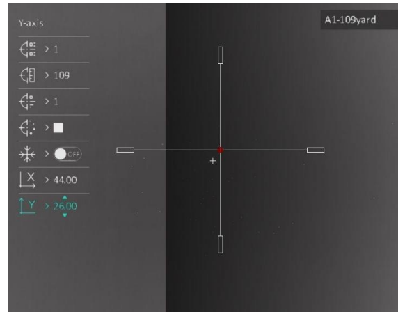
Abbildung 2-11 Nullstellung
