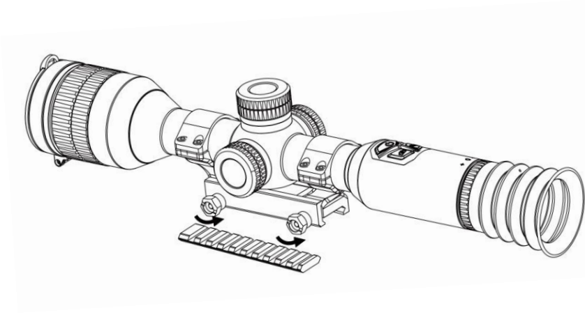
Figura 2-8 Aflojar los tornillos
