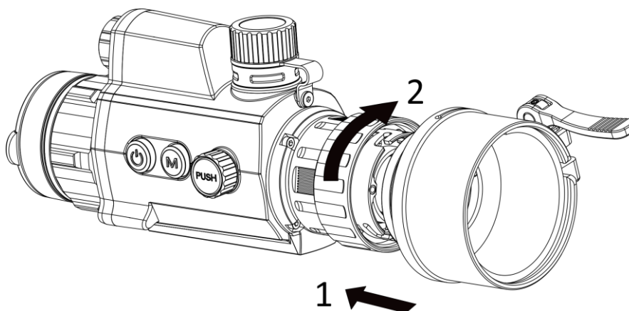
Figure 2-2 Installation de l'adaptateur
