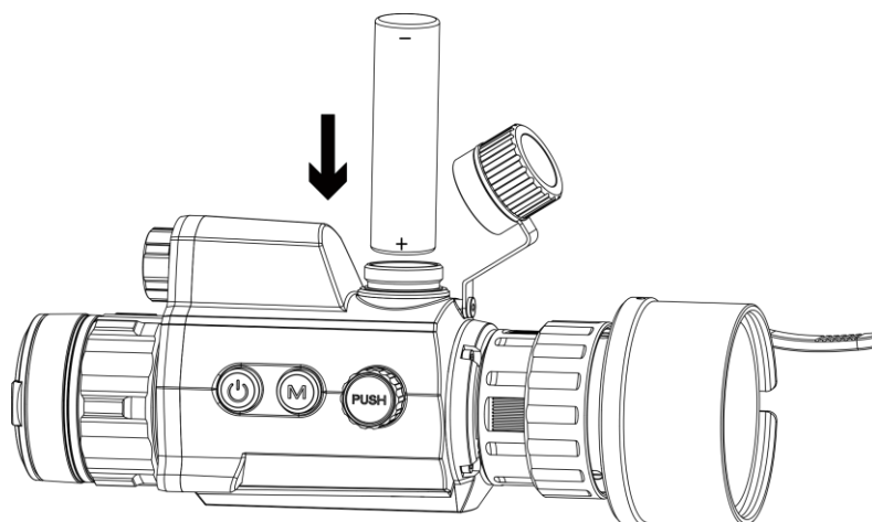
Figure 2-5 Installation de la batterie
