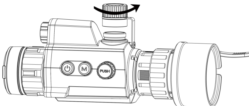
Figure 2-4 Ouverture du couvercle de la batterie
