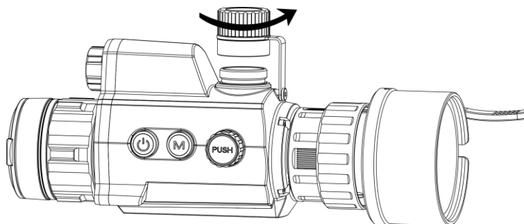
Obrázok 2-4 Otvorte kryt batérie
