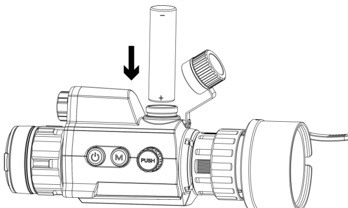
Obrázok 2-5 Inštalácia batérie
