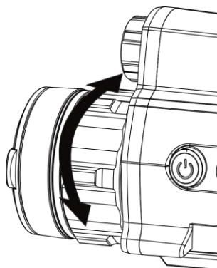
Obrázok 3-1 Nastavenie zaostrenia
