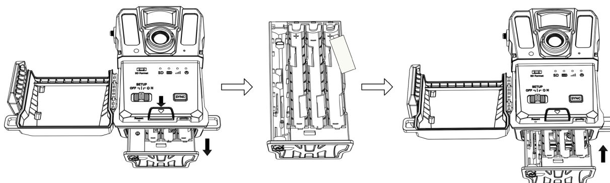
Obrázek 2-1 Vložení baterií
