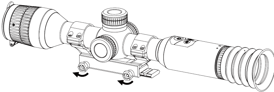
2-9. ábra: Csavarok meghúzása
