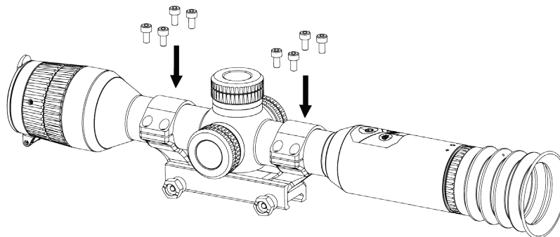
2-7. ábra: Csavarok meghúzása
