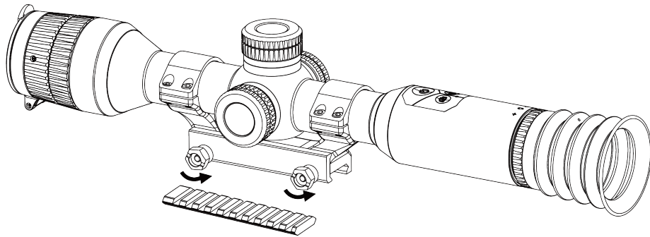
2-8. ábra: Csavarok kilazítása
