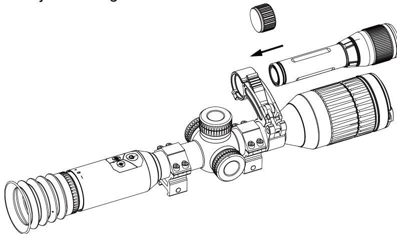
2-12. ábra: Az infravörös lámpa becsavarozása
