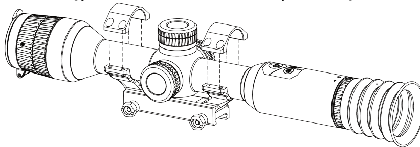
2-6. ábra: Az eszköz összekapcsolása a gyűrűvel
