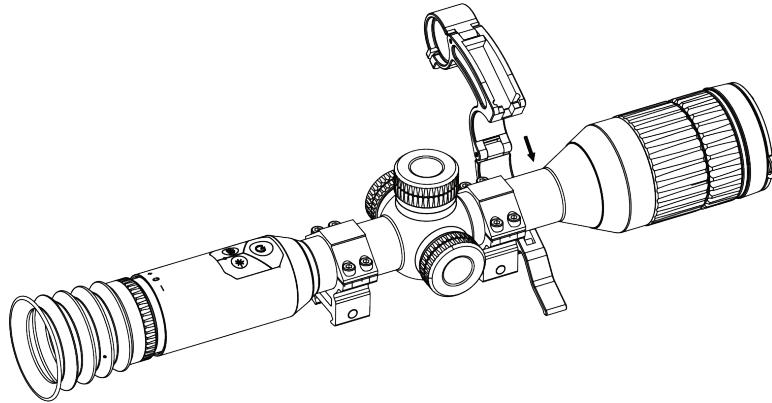
2-10. ábra: Az infravörös lámpa konzoljának felnyitása
