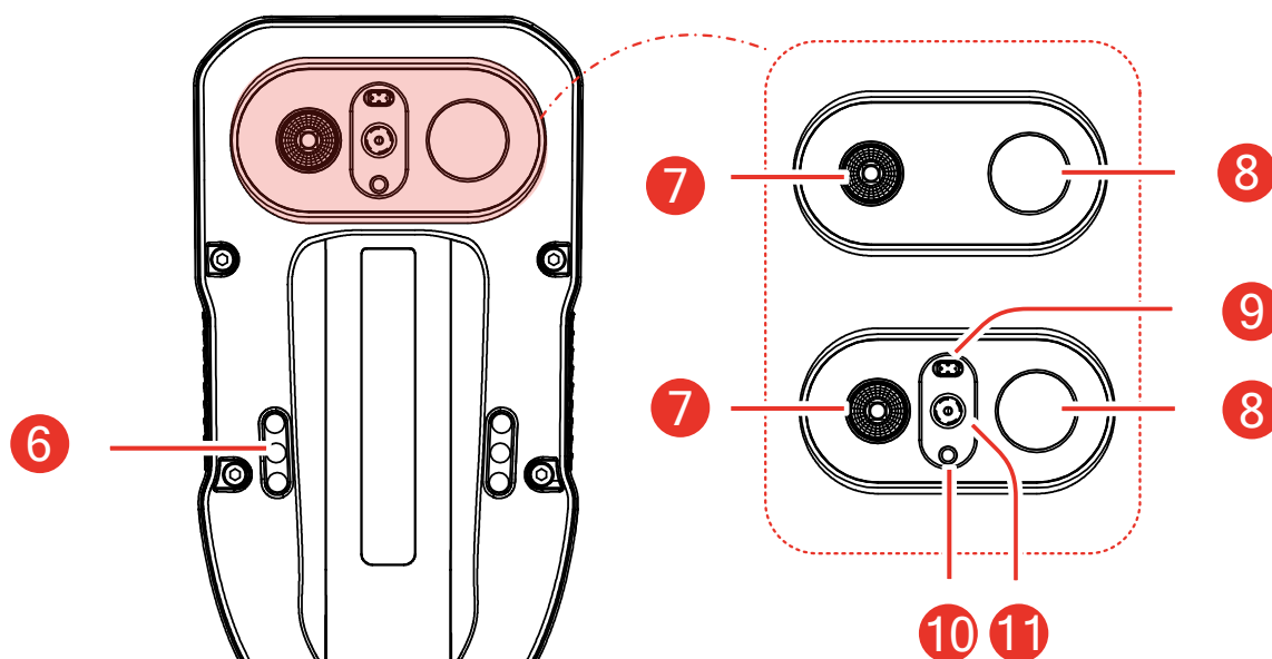
Rysunek 1-2 Wygląd (widok z tyłu)
