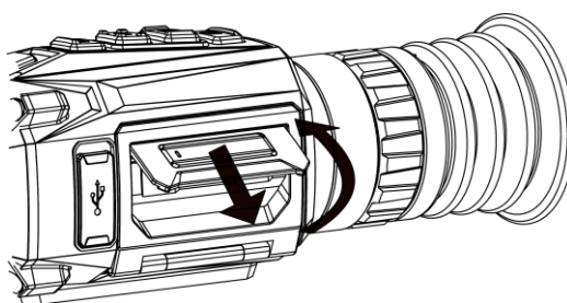
Figure 2-1 Retrait du couvercle du compartiment de la batterie
