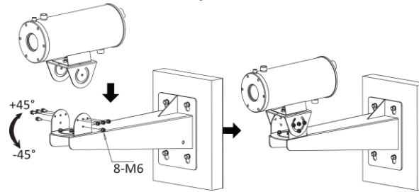
Afbeelding 3-7 De kantelhoek aanpassen
