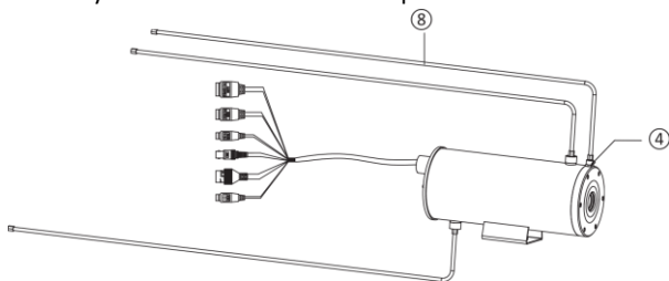
Obrázok 3-11 Inštalácia odprašovania
