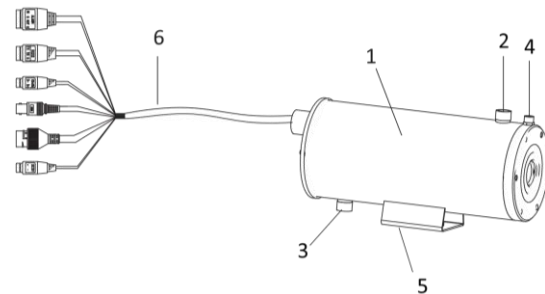
그림 2-1 외관
