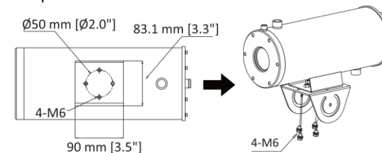
Рисунок 3-6. Установіть верхню частину поворотно-нахильного кронштейна на камеру
