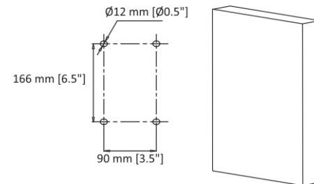
圖 3-1 在牆上鑽孔
