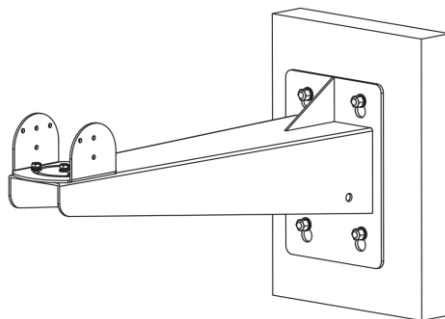
Рисунок 3-4. Установіть кронштейн
