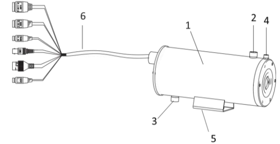
Şekil 2-1 Görünüm
