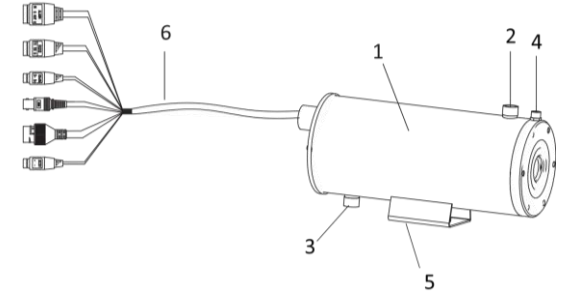
Figura 2-1 Aspeto
