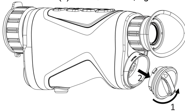
Figur 2-1 Løsne dekselet
