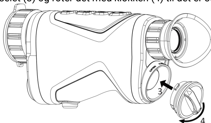
Figur 2-3 Stramme dekselet
