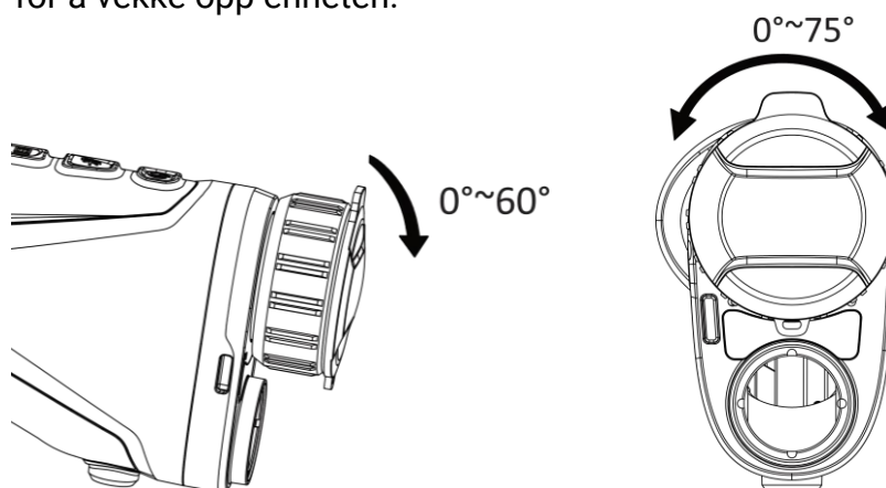
Figur 2-8 Vekk enheten
