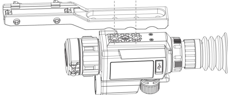
Figur 2-5 Sentrer installasjonshullene
