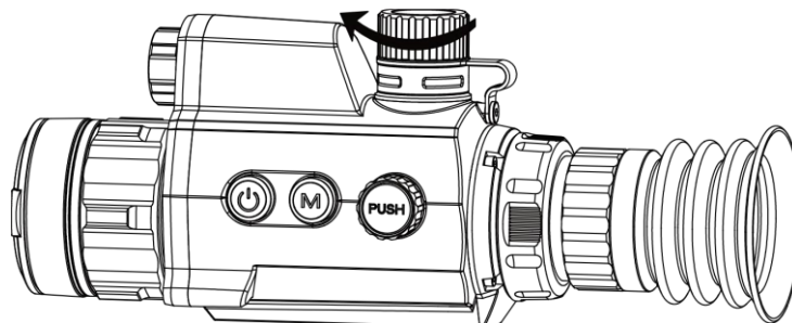
Figur 2-4 Lukk batteridekselet
