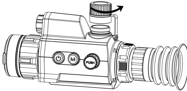
Figur 2-2 Åpne batteridekselet
