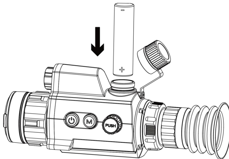
Figur 2-3 Sette inn batteriet
