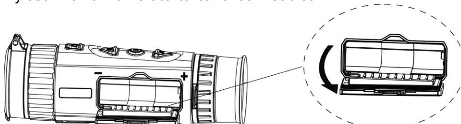
2-2. ábra: Nyissa ki az akkumulátortartó rekesz fedelét
