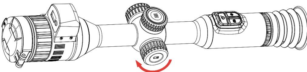
Obrázok 2-4 Uťahnite kryt
