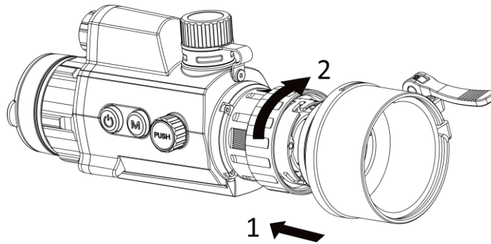
Abbildung 2-2 Adapter montieren
