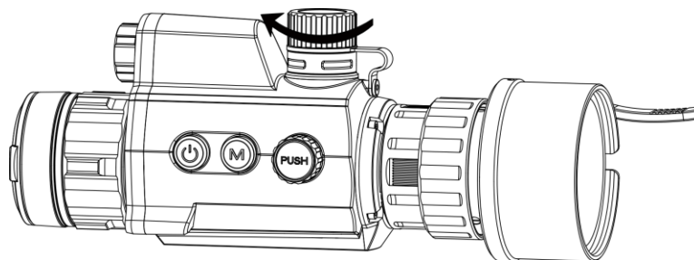
Abbildung 2-5 Batterieabdeckung schließen
