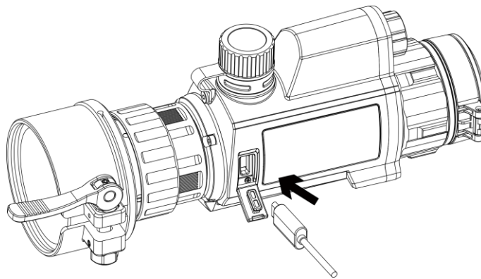
Abbildung 2-1 Kabelanschluss
