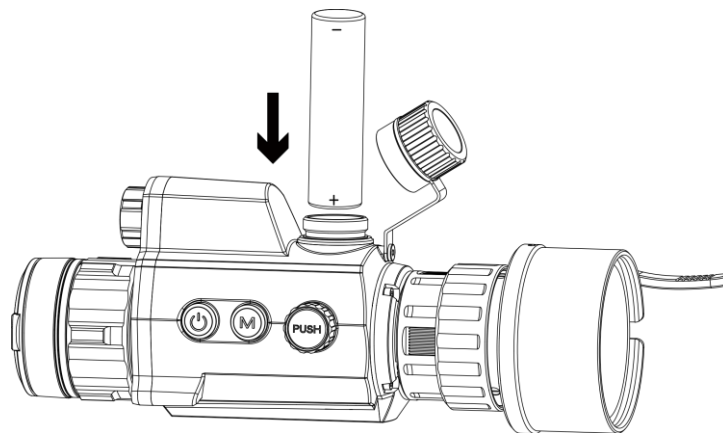
Abbildung 2-4 Akku einsetzen
