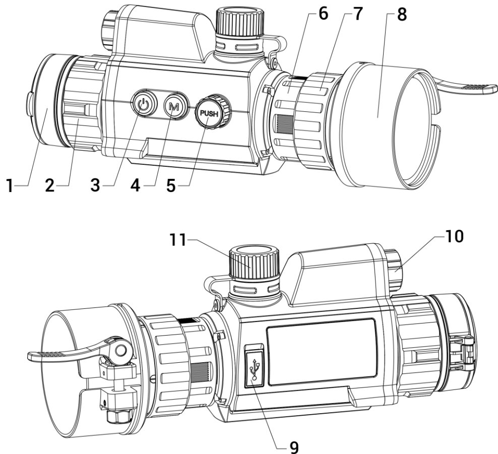
Abbildung 1-1 Gerät Erscheinungsbild
