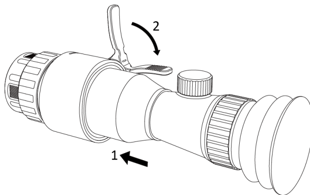
Abbildung 2-3 Tageslichtzielfernrohr montieren
