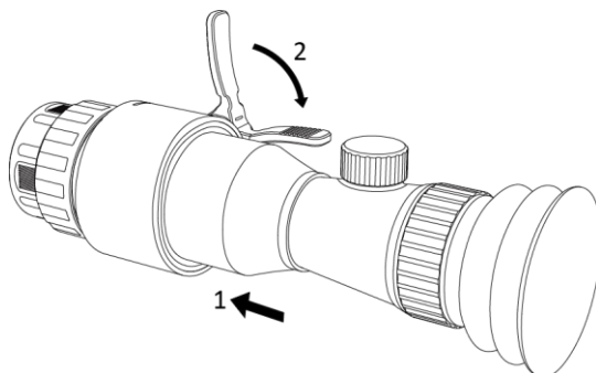
Figur 2-6 Montera dagsljussiktet
