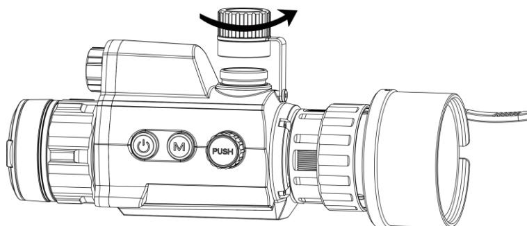
Obrázek 2-4 Otevření krytu bateriového prostoru
