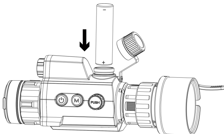
Obrázek 2-5 Vložení baterií
