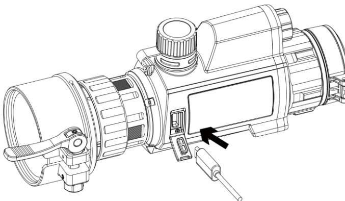
Obrázek 2-1 Zapojení kabelů
