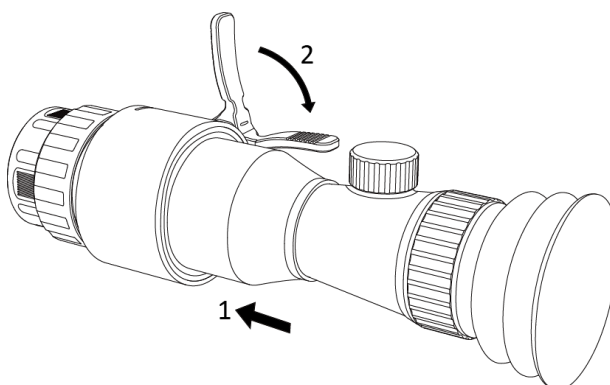
Obrázek 2-3 Montáž hledí pro denní světlo
