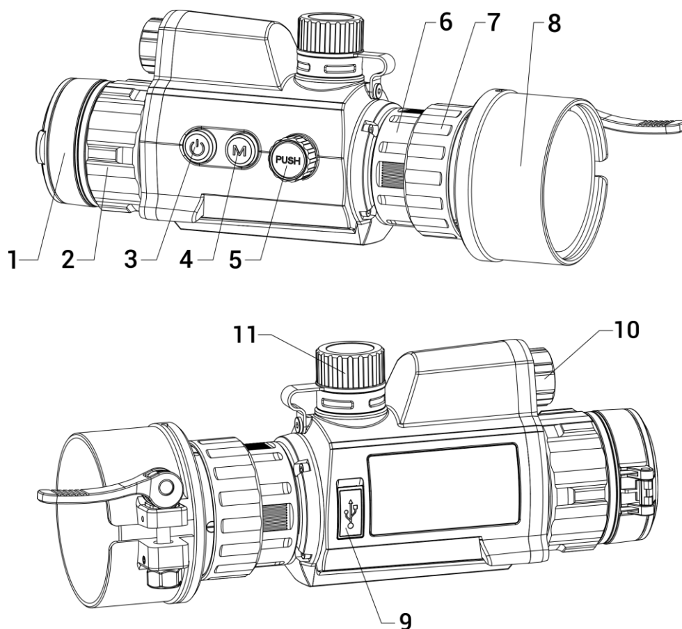
Obrázek 1-1 Vzhled zařízení
