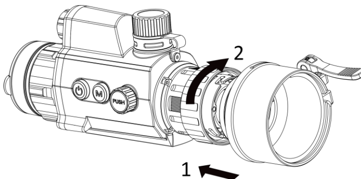
Obrázek 2-2 Montáž adaptéru
