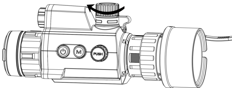
Obrázek 2-6 Uzavření krytu bateriového prostoru
