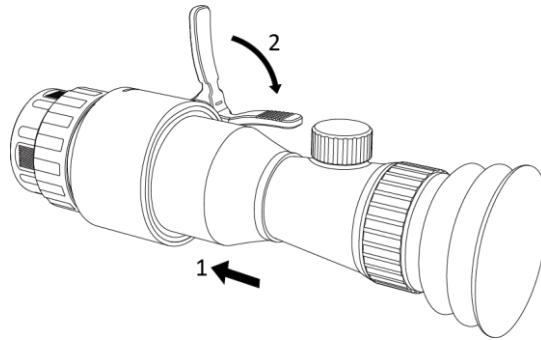
Figura 2-5 Instalación de la mira telescópica diurna
