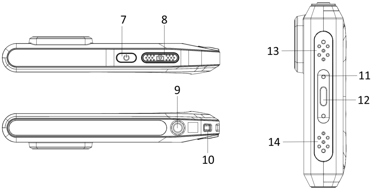
Abbildung 1-1 Aufbau
