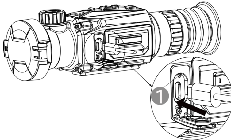
Abbildung 2-4 Kabelanschluss
