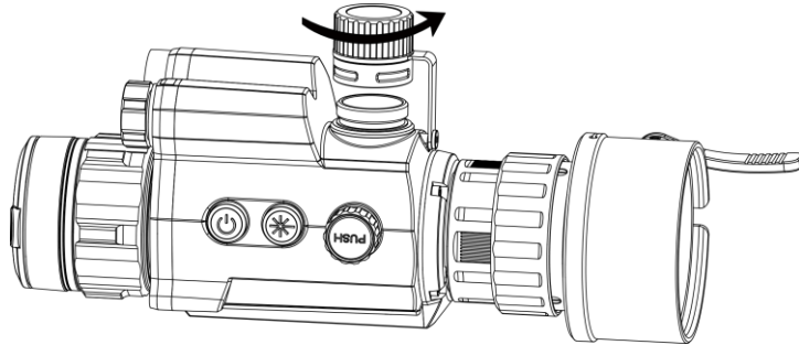
그림 2-3 배터리 커버 열기
