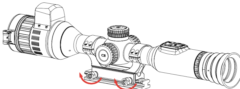
Figura 2-9 Serraggio delle viti
