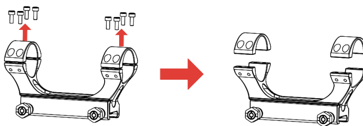
Figura 2-5 Apertura della parte superiore dell'anello
