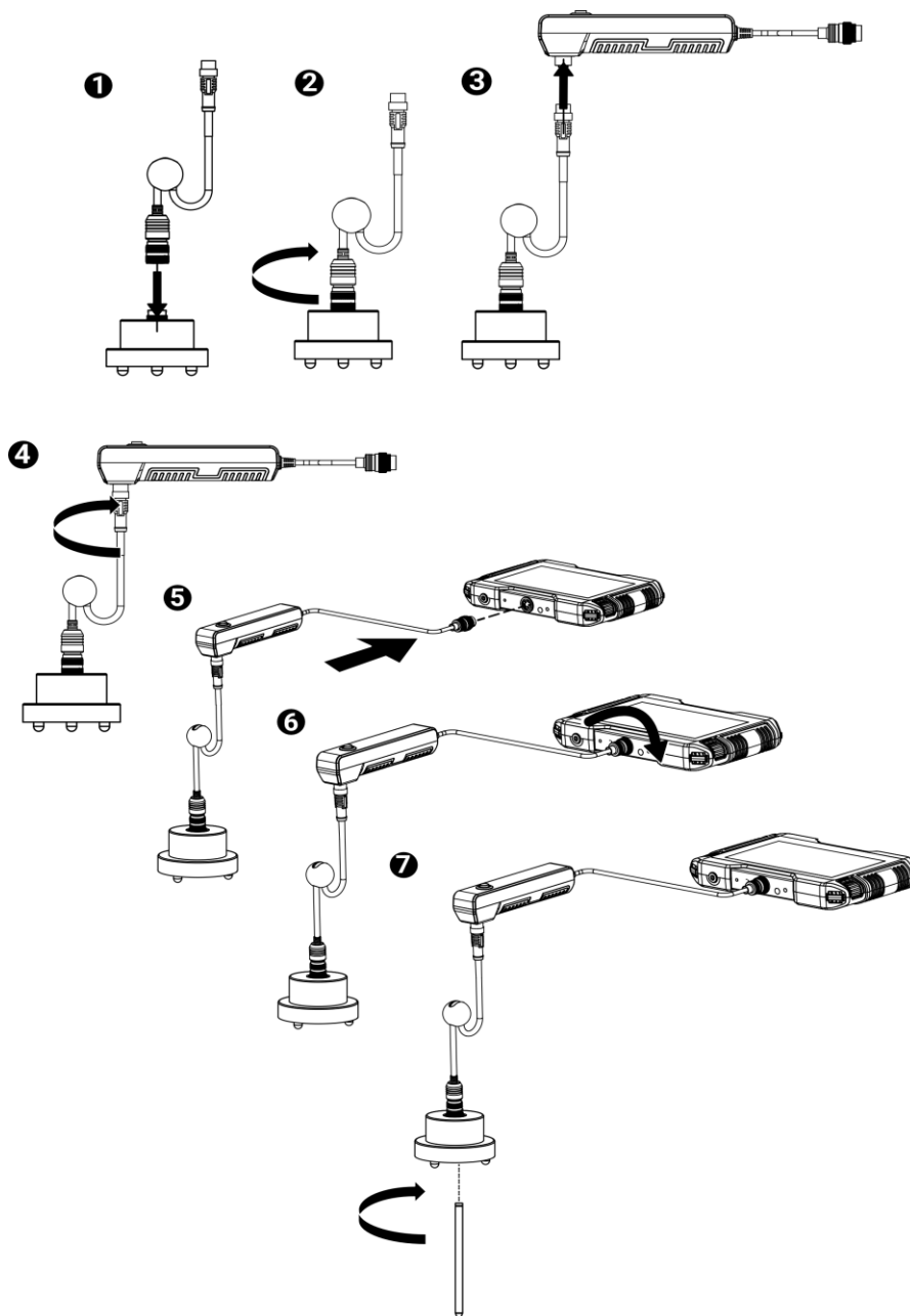
Figura 2-3 Montaggio del sensore esterno
