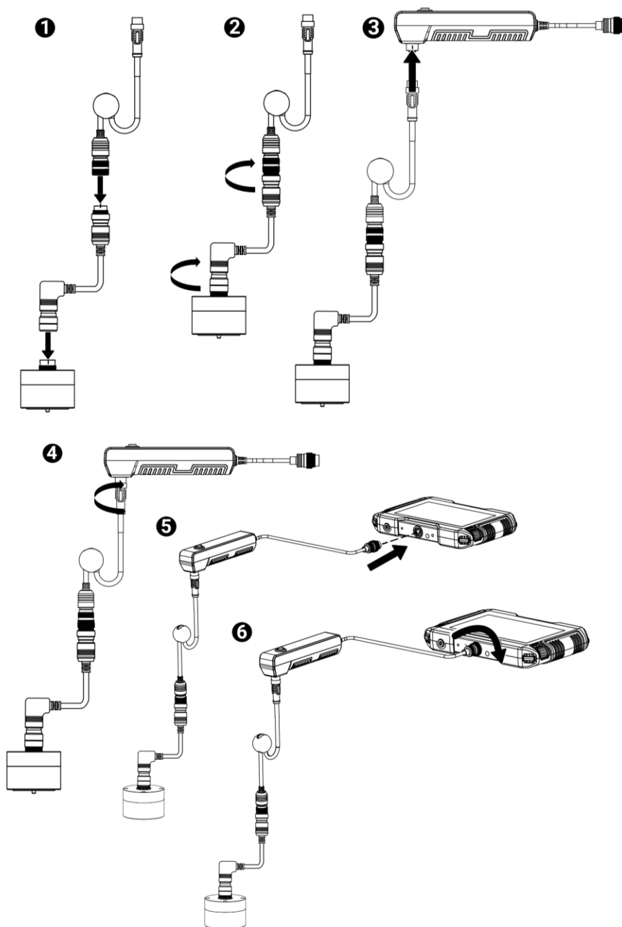
Figura 2-2 Montaggio del sensore portatile
