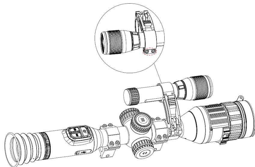
Figura 2-13 Fissaggio della torcia a infrarossi
