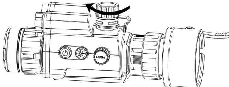
Figur 2-5 Lukk batterideksel
