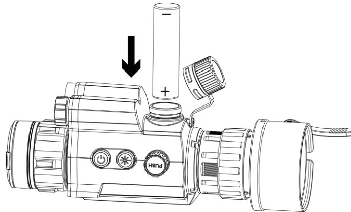
Figur 2-4 Installer batteri
