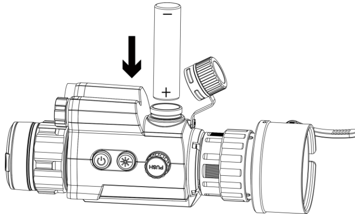
Abbildung 2-5 Akku einsetzen
