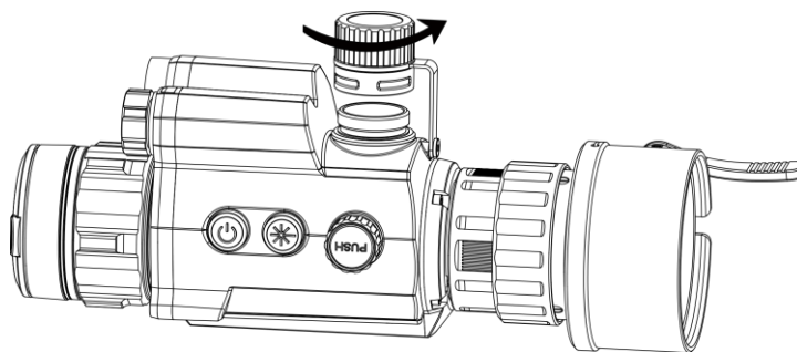
Abbildung 2-4 Batterieabdeckung öffnen
