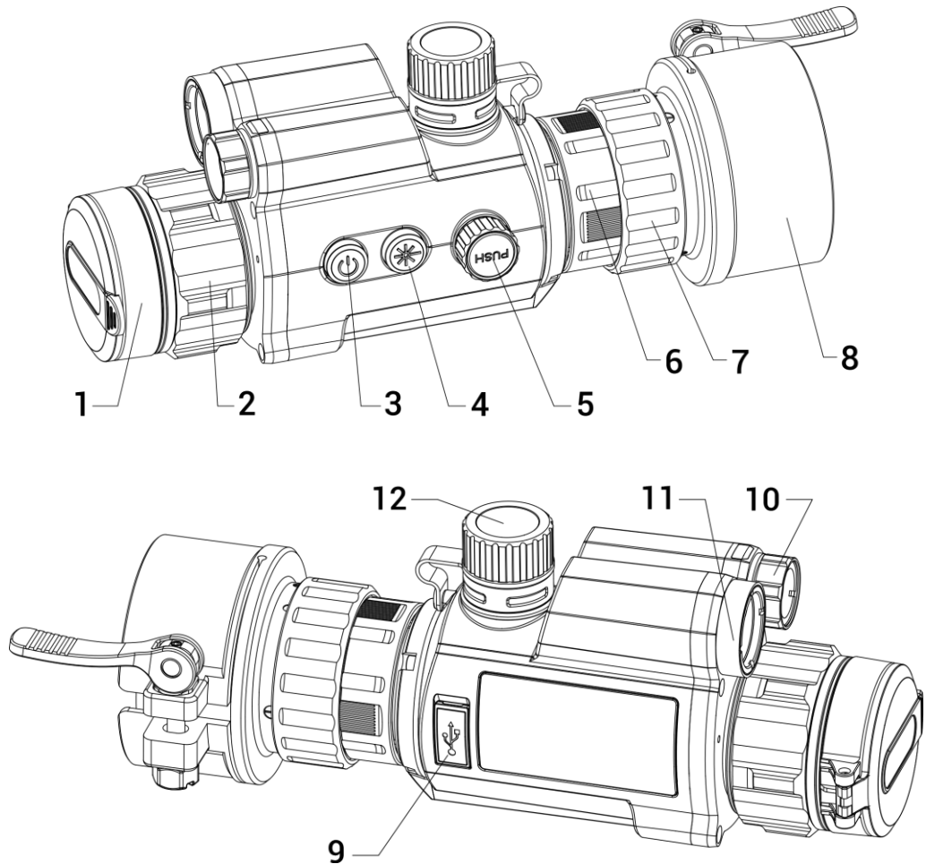
Abbildung 1-1 Gerät Erscheinungsbild
