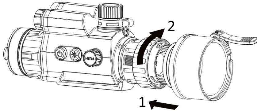
Abbildung 2-2 Adapter montieren
