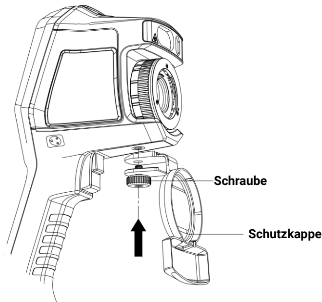
Abbildung 2-5 Schutzabdeckung befestigen
