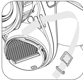
Figure 2-5 Enfilage de la sangle de cou dans les points de fixation
