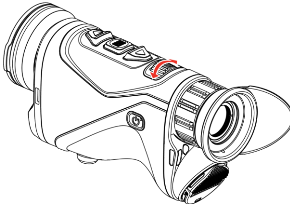
Figure 3-2 Réglage de la mise au point
