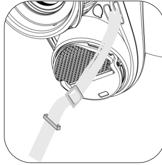
Figure 2-7 Enfilage de la sangle de cou dans le support de sangle
