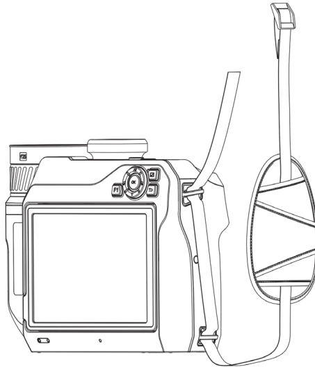
Abbildung 2-4 Handschlaufe durch die Befestigungspunkte einfädeln
