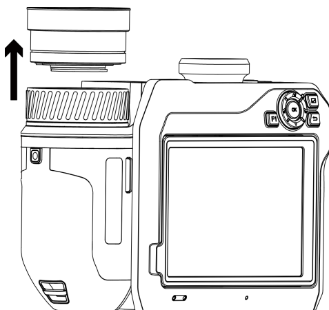
Abbildung 2-7 Objektiv entfernen
