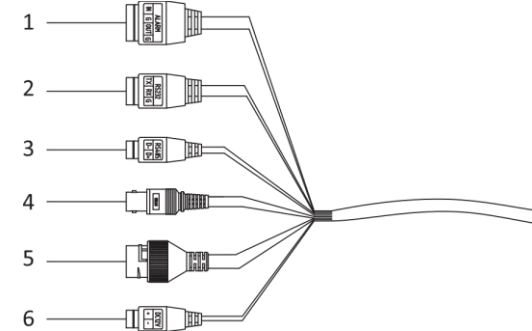
Figura 2-2 Cavi della telecamera
