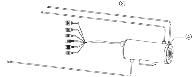
Imagen 3-11 Instalación de retirada del polvo
