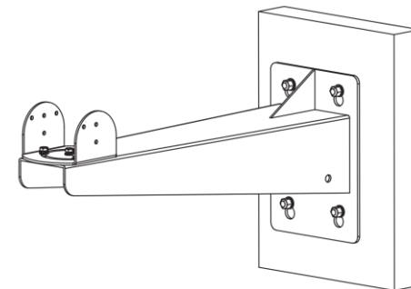
Obrázok 3-4 Nainštalujte konzolu
