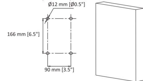
Imagen 3-1 Taladrar agujeros en la pared
