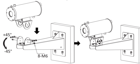
Afbeelding 3-7 De kantenhoek aanpassen
