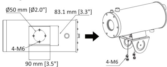
Afbeelding 3-6 De bovenkant van het PT-verbindingsstuk installeren op de camera
