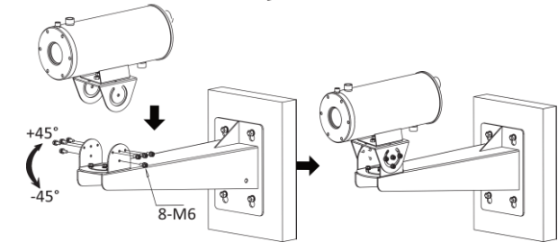
Abbildung 3-7 Neigungswinkel anpassen
