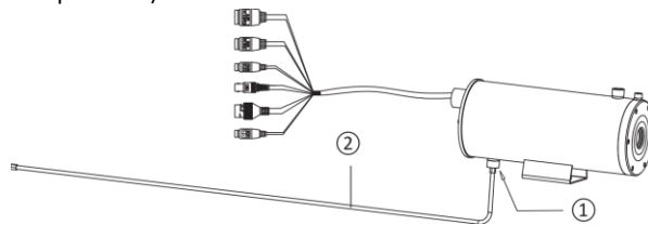
Рисунок 3-8. Присоединение труб для воздушного охлаждения
