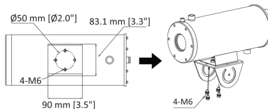
Rysunek 3-6 Mocowanie górnej części uchwyty uchylnej do kamery
