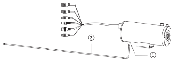
Obrázek 3-8 Připojení trubky pro chlazení vzduchem
