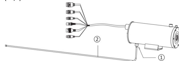
Rysunek 3-8 Podłączanie przewodu doprowadzającego powietrze chłodzące
