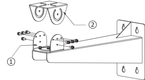
Figura 3-3 Disassemblare il giunto snodato
