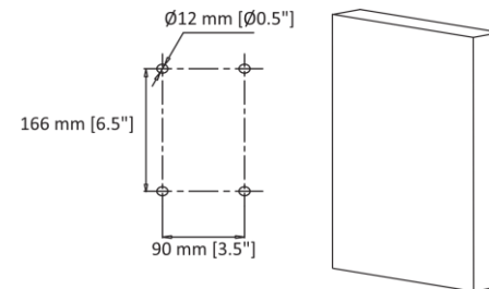
圖 3-1 在牆上鑽孔
