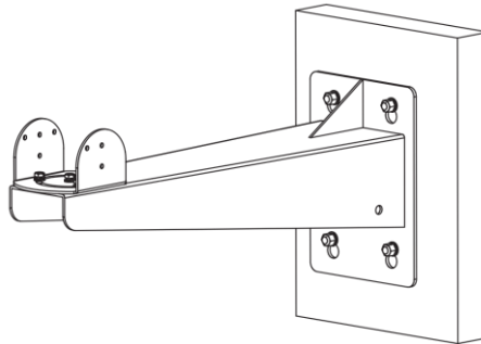
Рисунок 3-4. Установіть кронштейн
