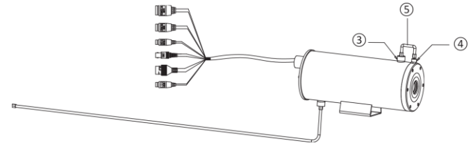
図 3-9 防塵機構の取り付け
