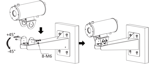
Şekil 3-7 Eğim Açısını Ayarlayın
