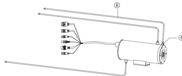
그림 3-11 방진 설치
