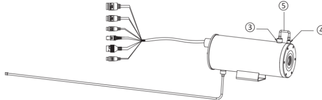
Abbildung 3-9 Entstaubende Installation
