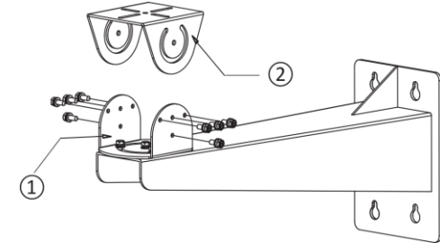
Afbeelding 3-3 Het PT-verbindingsstuk demonteren
