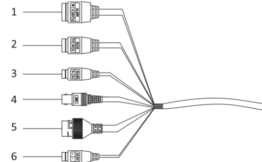
Rysunek 2-2 Przewód kamery
