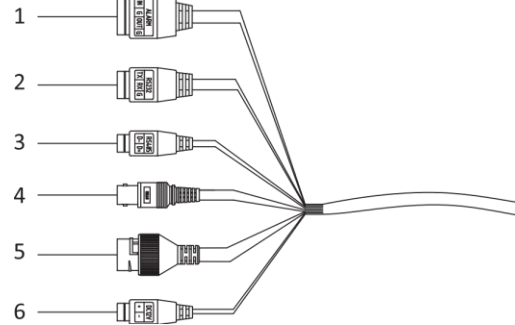
Рисунок 2-2. Кабелі камери
