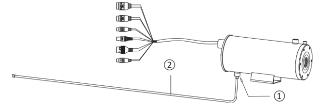
Afbeelding 3-8 Buisaansluiting voor luchtkoeling
