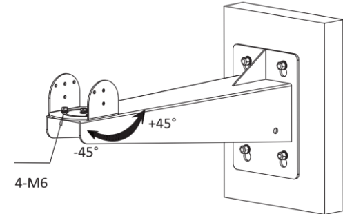
図 3-5 パン角度の調整
