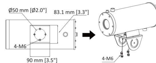
Figura 3-6 Instale o topo da junta PT com a câmera
