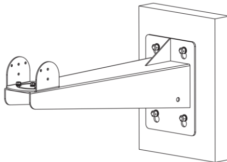
Рисунок 3-4. Установка кронштейна
