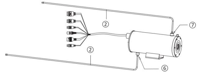
図 3-10 水冷用配管接続
