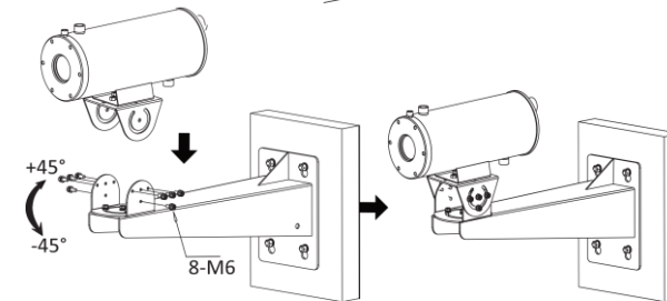
Figura 3-7 Ajuste o ângulo de inclinação
