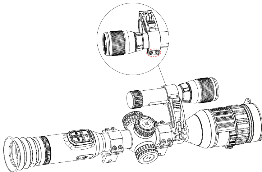
그림 2-13 IR 토치 고정
