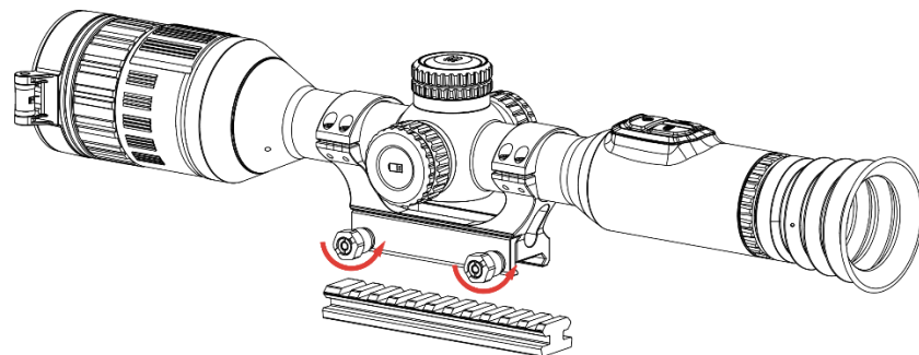
그림 2-8 나사 풀기
