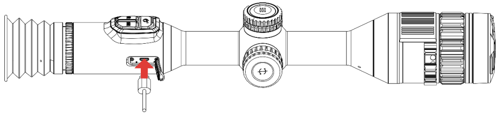
그림 2-1 케이블 연결
