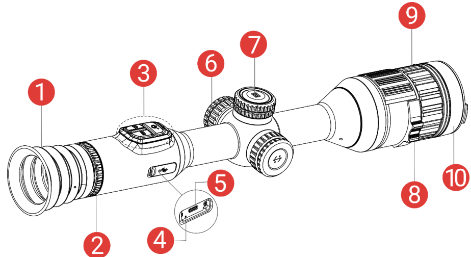
그림 1-1 외관
