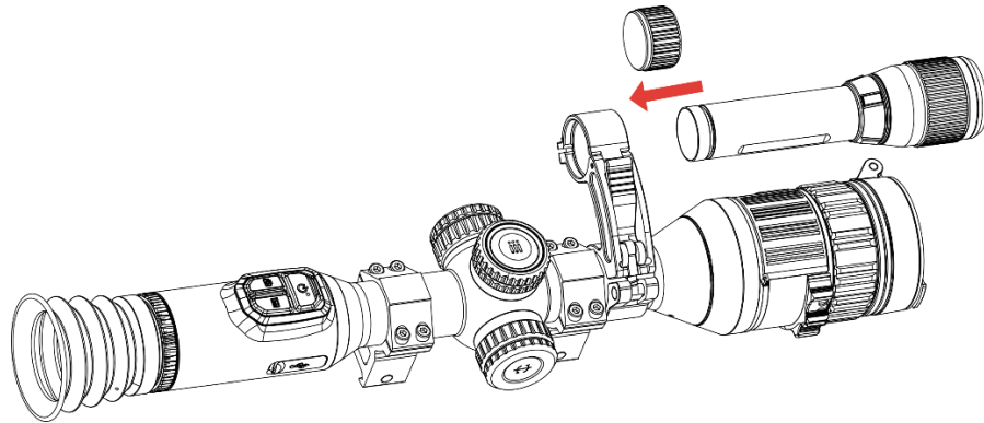
그림 2-12 IR 토치 끼우기
