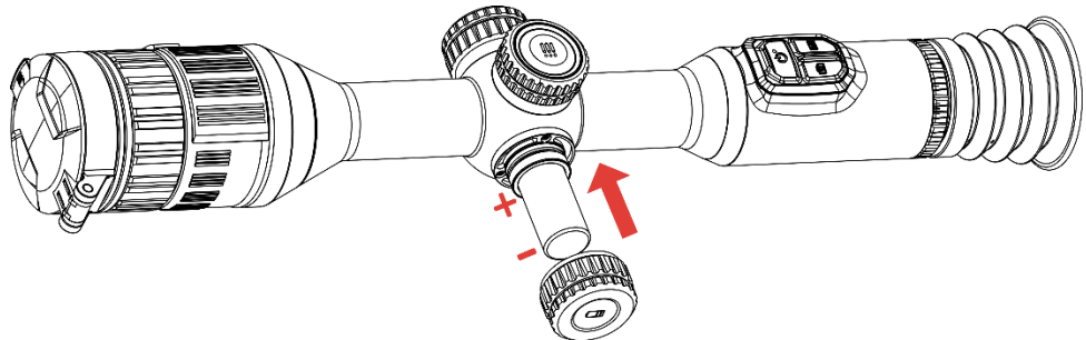
그림 2-3 배터리 삽입
