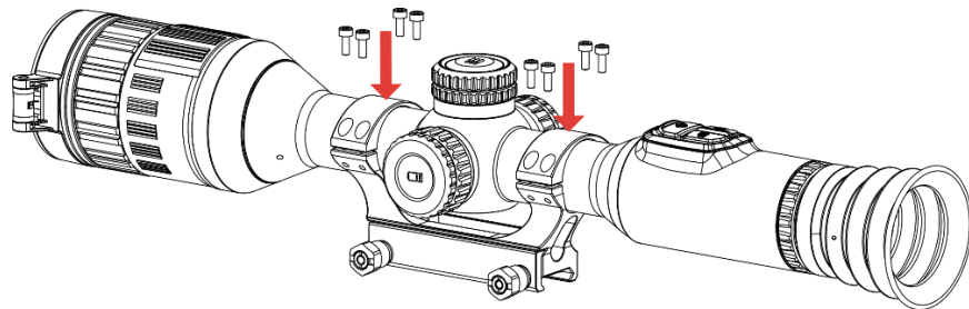
그림 2-7 나사 조이기
