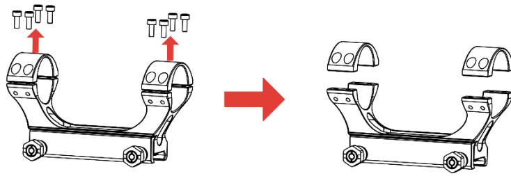
그림 2-5 링 상단 나사 풀기
