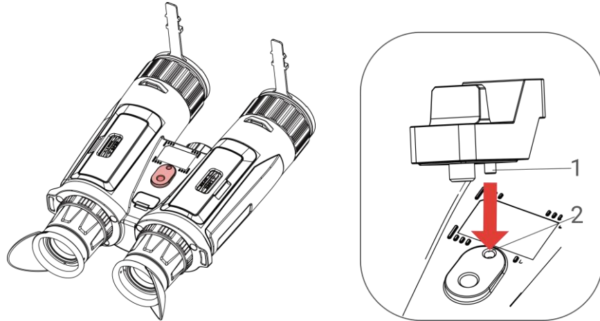
Abbildung 2-11 Den Führungsstift einsetzen
