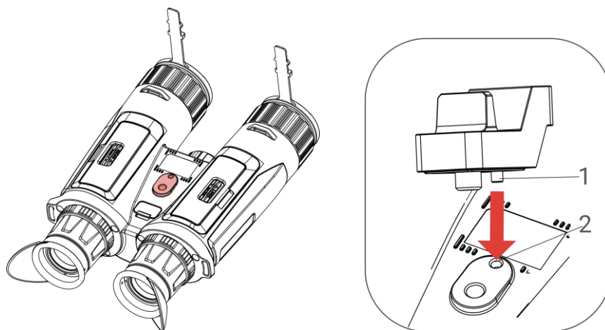
Obrázek 2-11 Vložení sloupku
