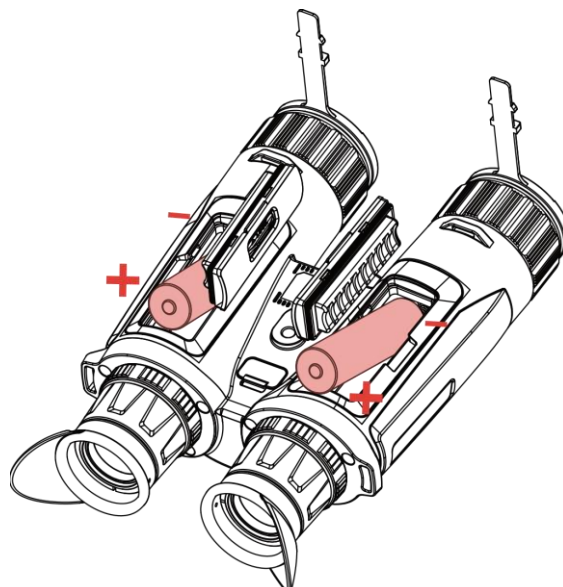
Obrázek 2-2 Vkládání baterií
