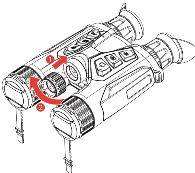
Obrázek 2-6 Montáž přísvitu
