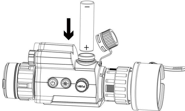
그림 2-5 배터리 설치
