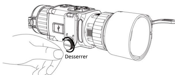
Figure 2-2 Desserrage de la vis à main
