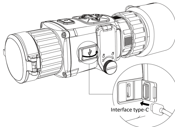
Figure 2-1 Interface du câble
