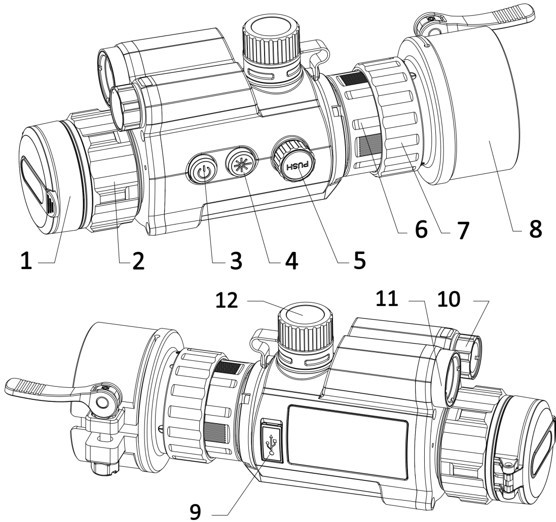
Figura 1-1 Aspecto del dispositivo
