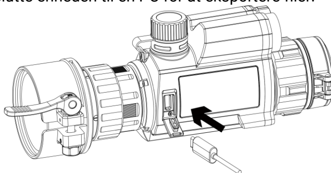
Figur 2-1 Kabeltilslutning
