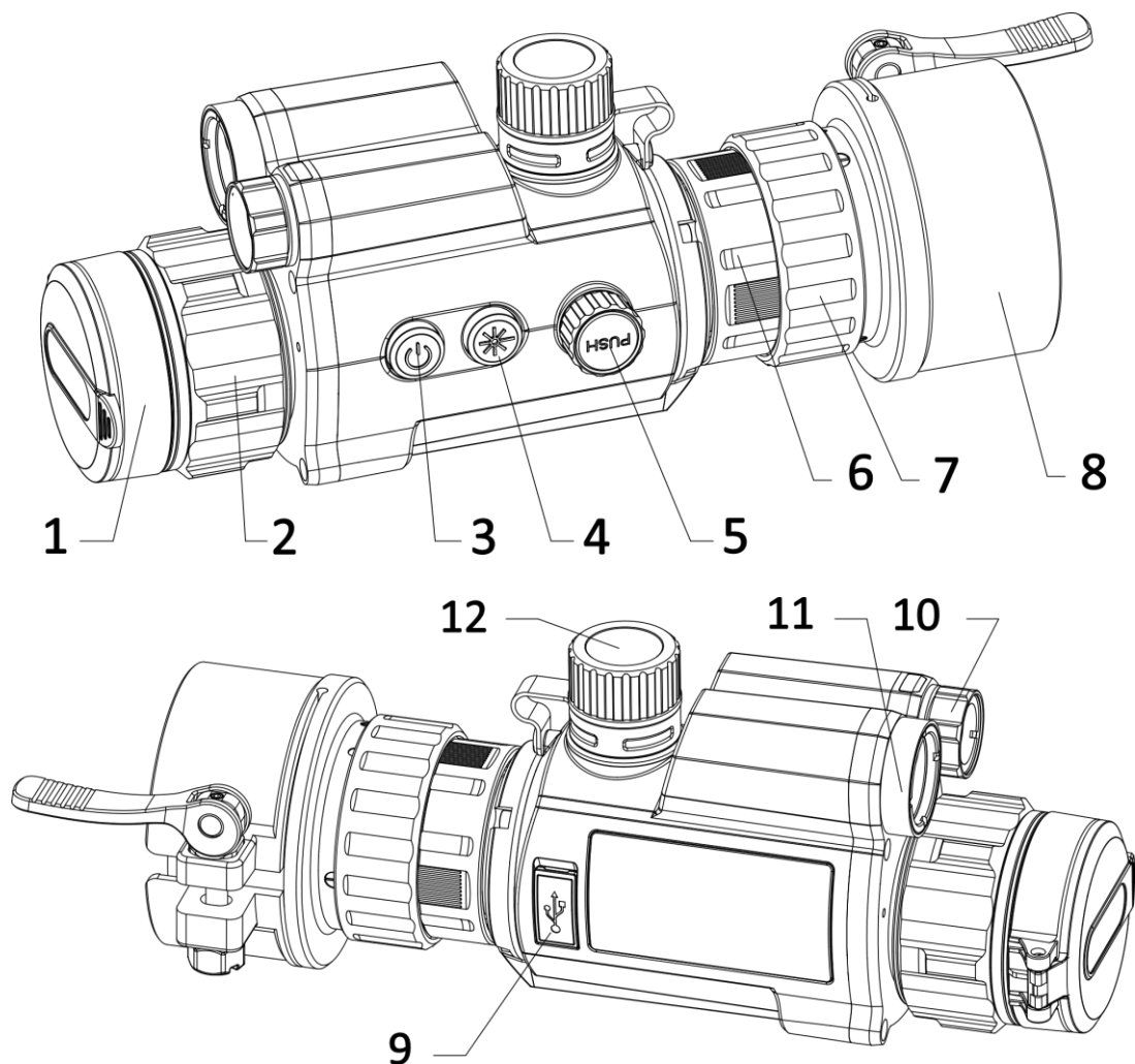
Figur 1-1 Enhedens udseende
