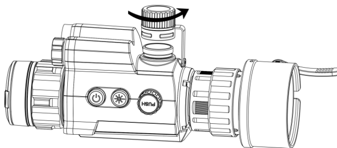
Figur 2-3 Åbn batteridækslet
