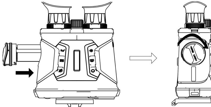
Abbildung 2-3 Akkufach einsetzen
