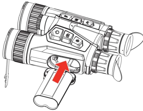
Gambar 2-2 Pasang Baterai
