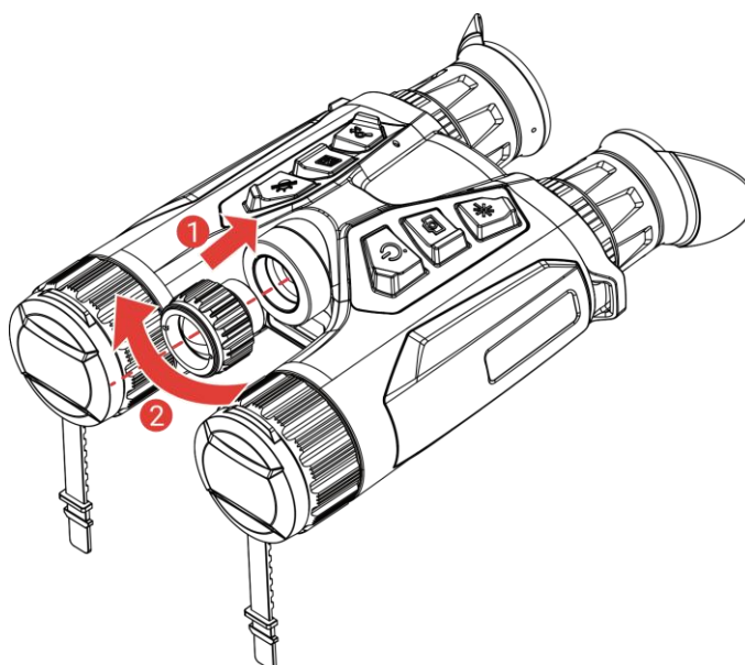
Obrázok 2-6 Upevnenie osvetľovača
