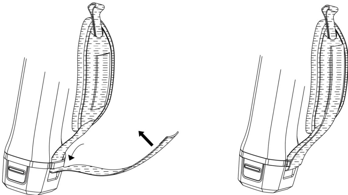
Abbildung 2-4 Den unteren Teil der Handschlaufe befestigen
