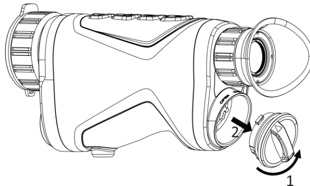
그림 2-1 커버 풀기
