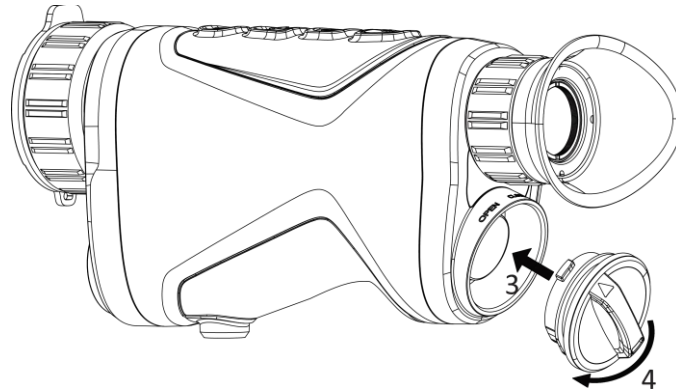
그림 2-3 커버 조이기
