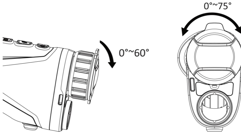
그림 2-8 장비 깨우기
