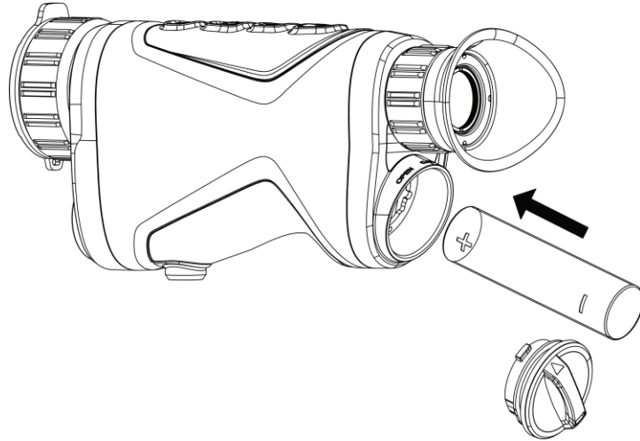
그림 2-2 배터리 설치
