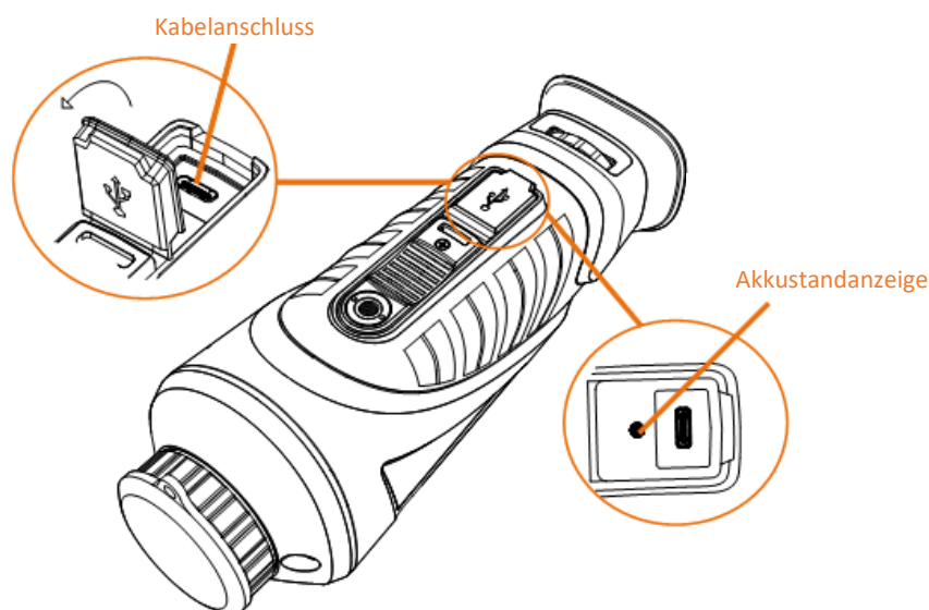
Abbildung 2-1 Kabelanschluss
